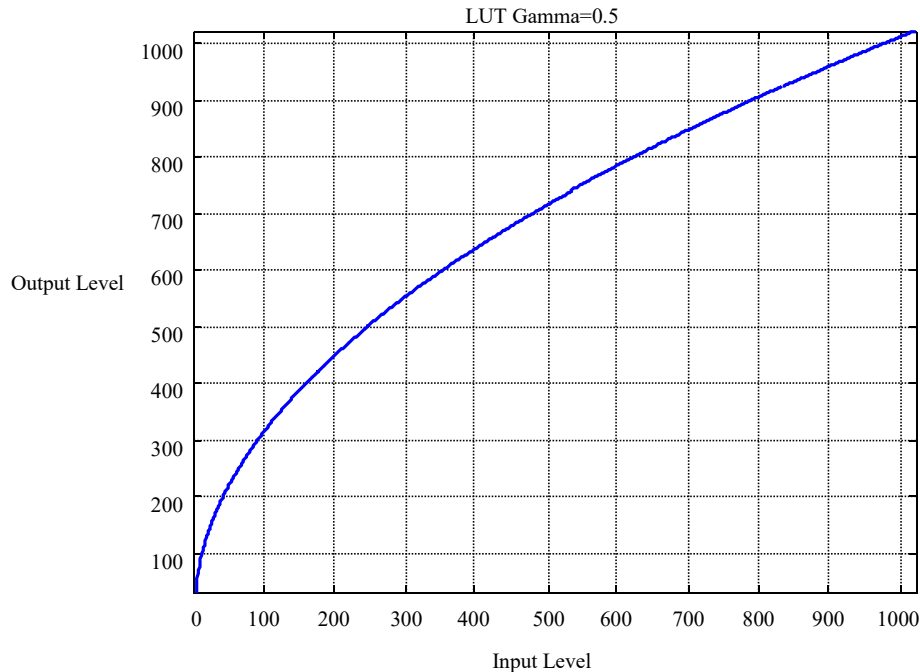
图 26 Gamma=0.5 对应的查找表
