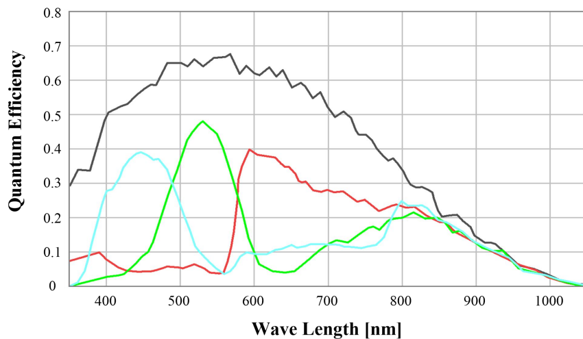
图 4 相机光谱响应
