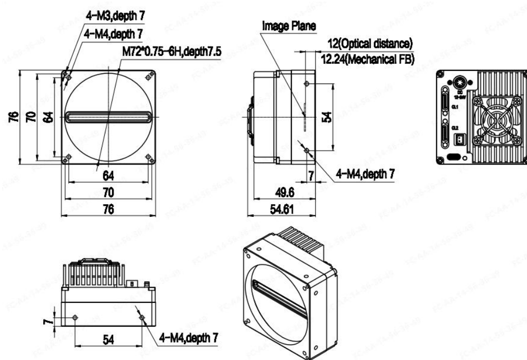
图 5 相机机械尺寸
