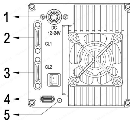
图 6 相机外部接口
