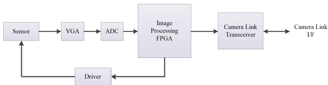
图 2 相机内部实现结构
