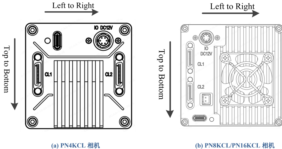
图 14 相机扫描方向
