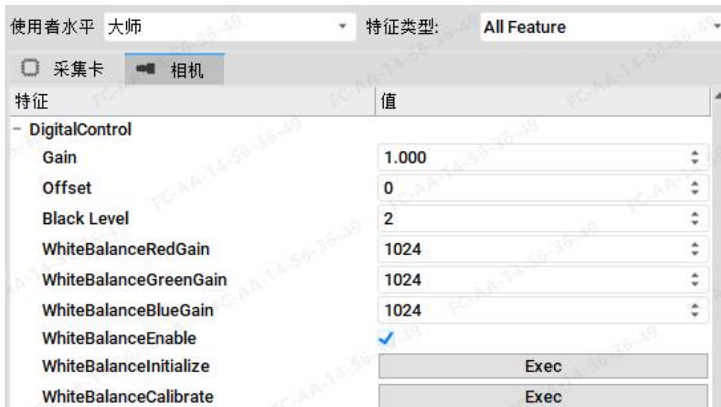
图 34 数字控制类别
