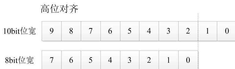
图 24 数据格式
