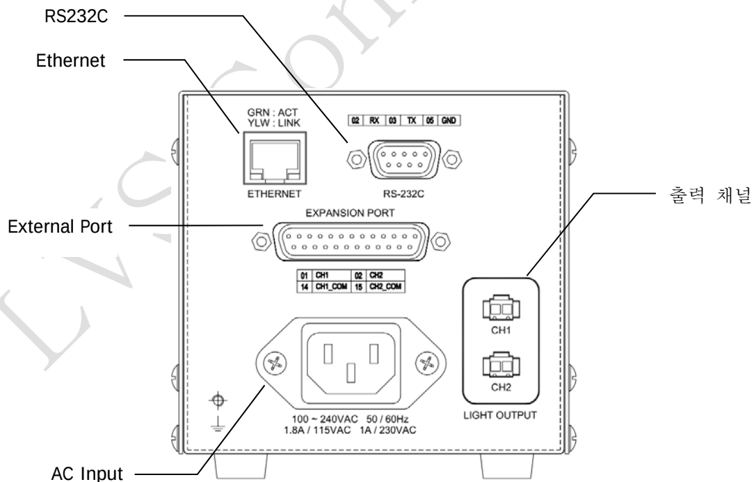
< EN-02 Series 후면부 >
