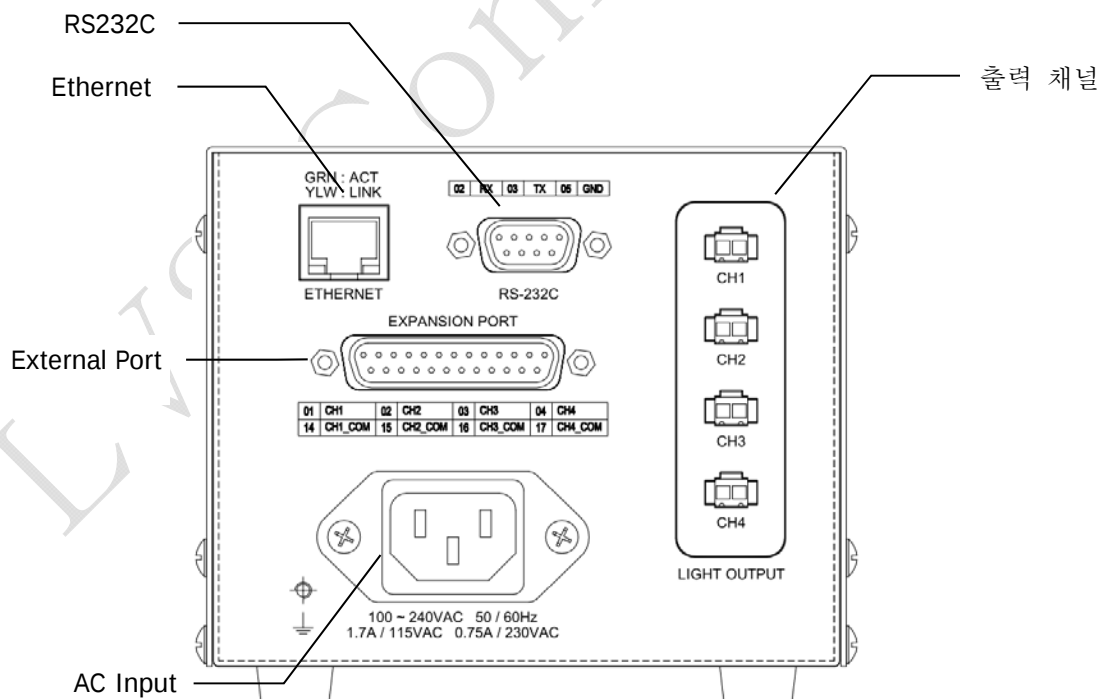
< EN-04 Series 후면부 >
